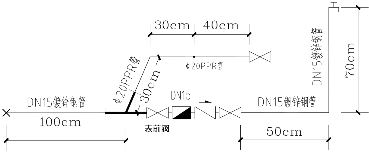
安装示意图:
